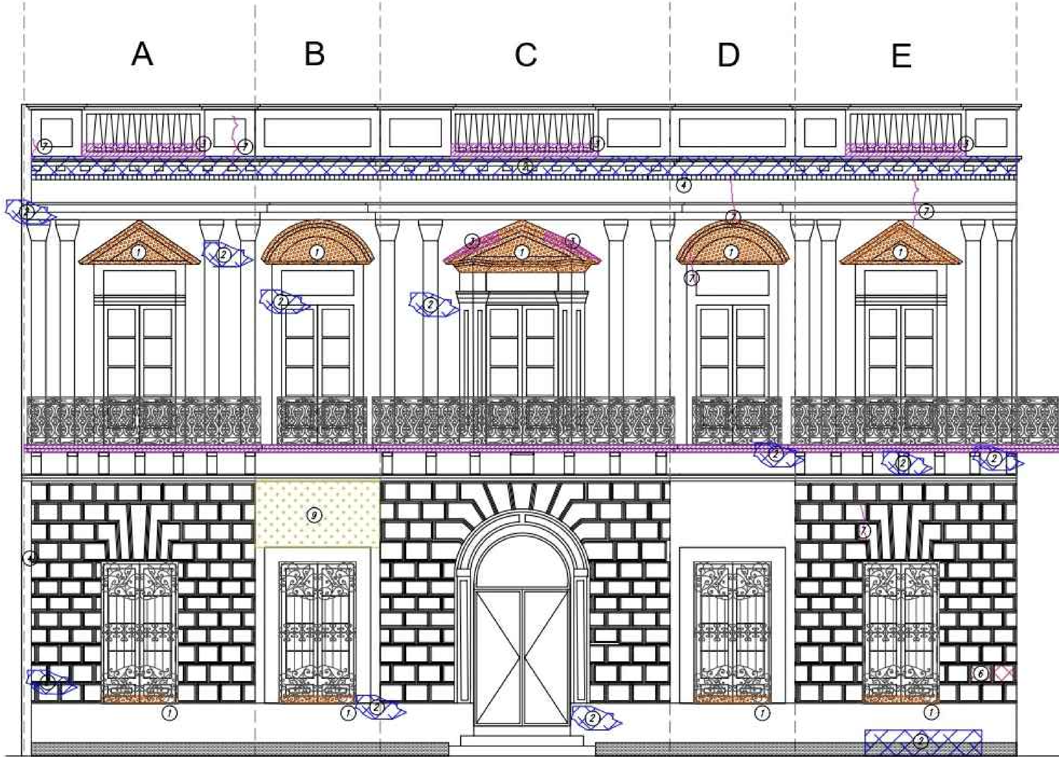
PATOLOGÍAS FACHADA SOBRE PLAZOLETA
